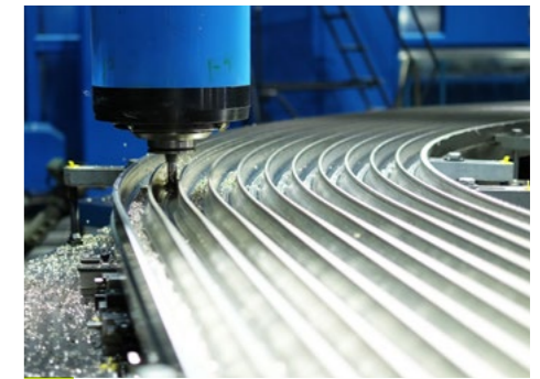
Fabrication série de 35 plaques radiales pour ITER
