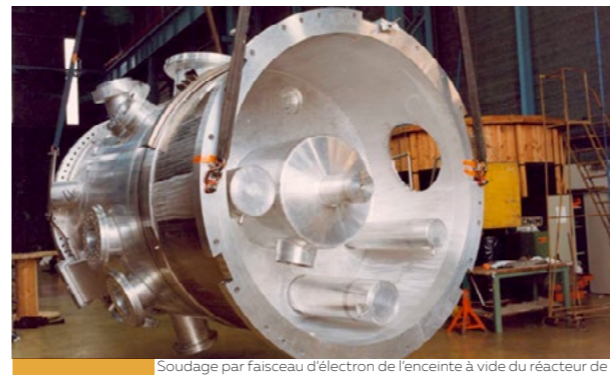
Soudage par faisceau d'électron de l'enceinte à vide du réacteur de la source expérimentale de neutrons Heinz Maier-Leibnitz (FRMI)
